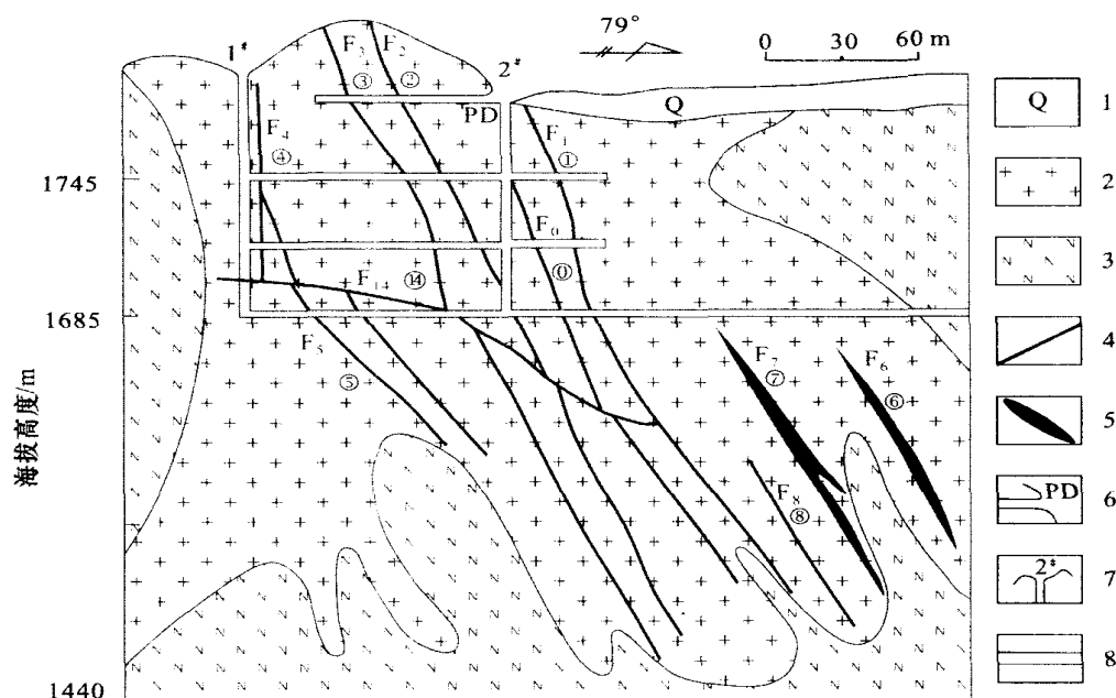
图4 I号埃达克岩体剖面控矿断裂与矿体形态图(据张照志,1999)
