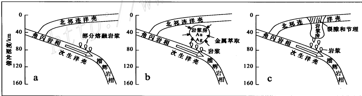
图 3 黑石山埃达克岩成矿模式图
