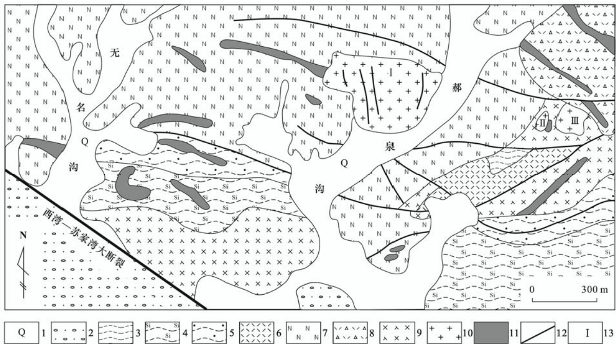
图 2 黑石山区域地质简图(据王光宁,1999)
