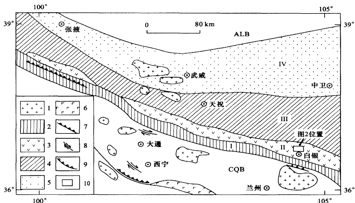
图1 北祁连大地构造简图(据许志琴,1997)
