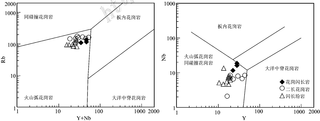
图 9 258 高地金矿区侵入岩构造判别图解(据 Pearce, 1996)
