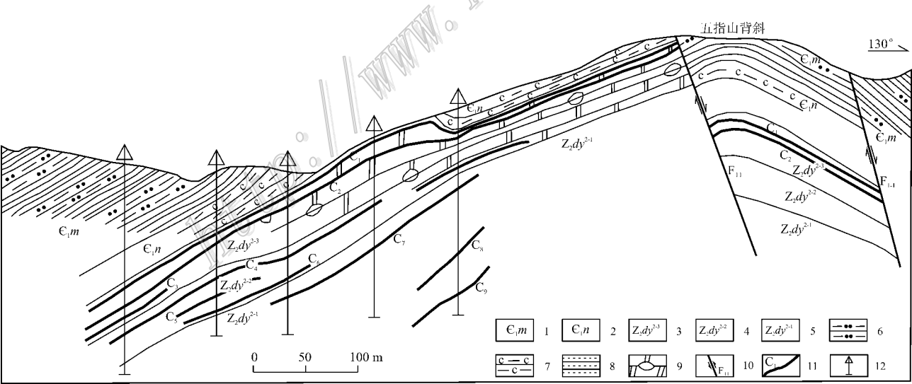
图 4 杜家桥铅锌矿床 6 号勘探线剖面图(据谭华等, 2012 修改)
