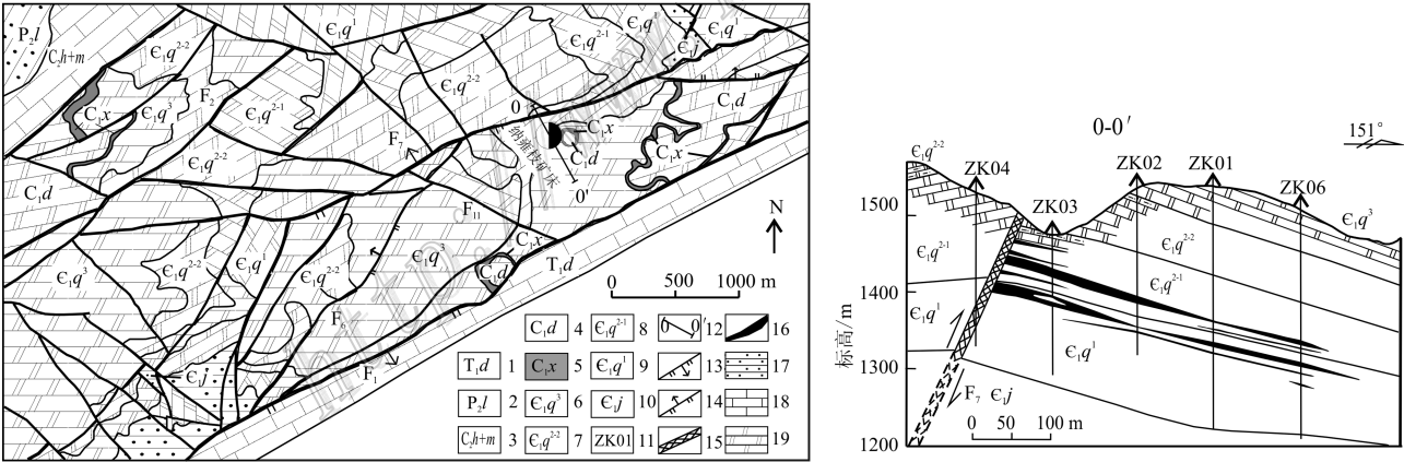
图 3 那雍枝矿床地质及 0 号剖面图
