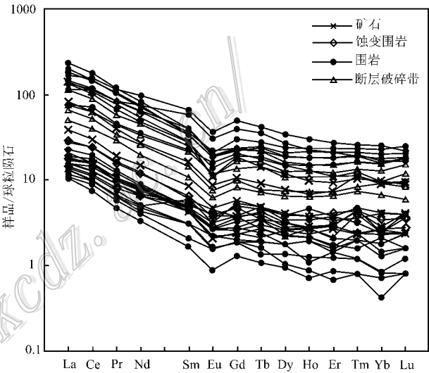
图 5 纳雍枝矿床稀土元素配分模式图
