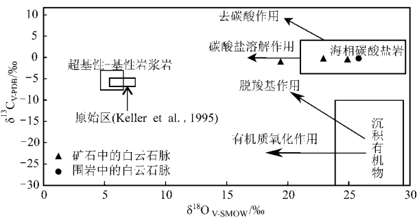
图 7 纳雍枝铅锌矿床 \delta^{13}\text{C}_{\text{V-PDB}}-\delta^{18}\text{O}_{\text{V-SMOW}} 图解(底图据袁波等,2014 修改 数据来源陈国勇等,2015)
