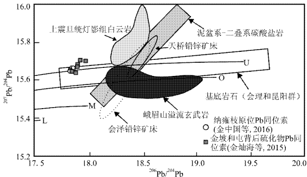
图 8 五指山地区铅锌矿床与地层沉积岩和基底岩石以及会泽和天桥的 ^{207}\text{Pb}/^{204}\text{Pb}-^{206}\text{Pb}/^{204}\text{Pb} 对比图解(据金中国等,2016 修改)上地壳(U)、造山带(O)、地幔(M)和下地壳(L)
