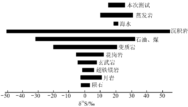
图 6 纳雍枝铅锌矿床硫化矿石硫同位素组成直方图
