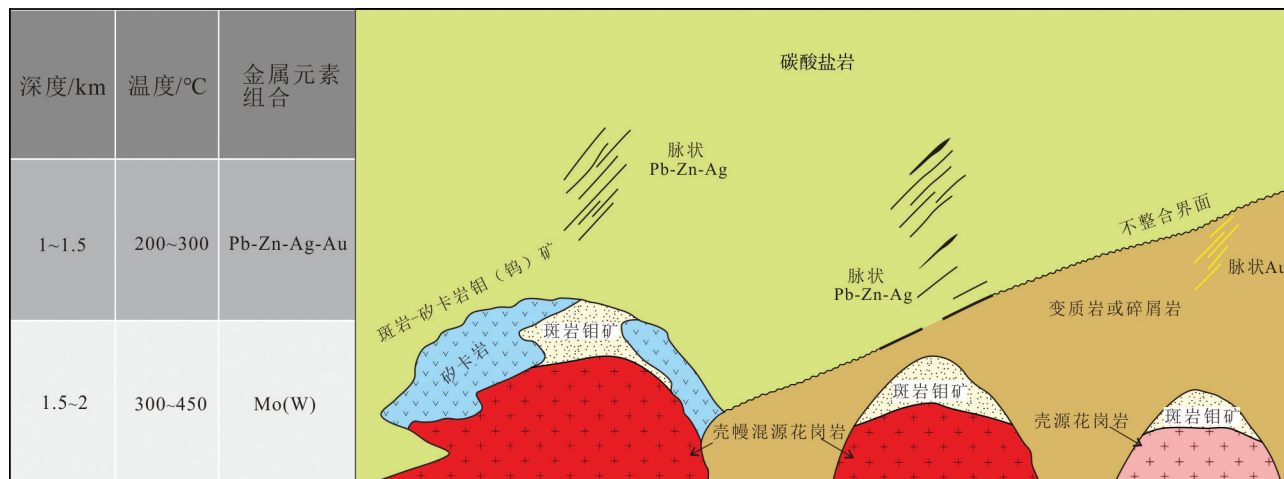
图1 斑岩-矽卡岩矿-远接触带脉状铅锌银矿模型(据毛景文等,2006修改)
