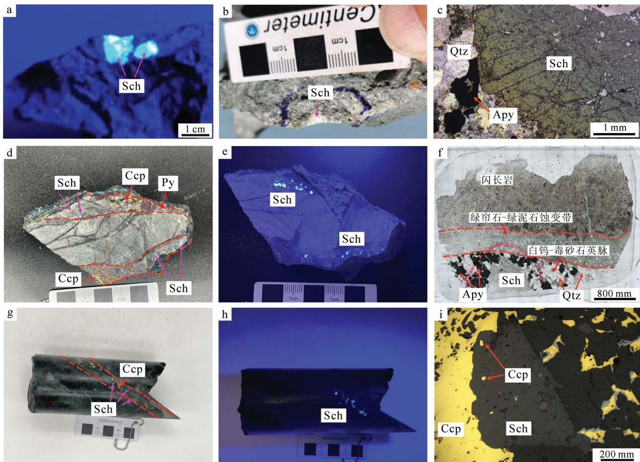
图2 莲花山矿区典型白钨矿矿石和显微镜下特征
